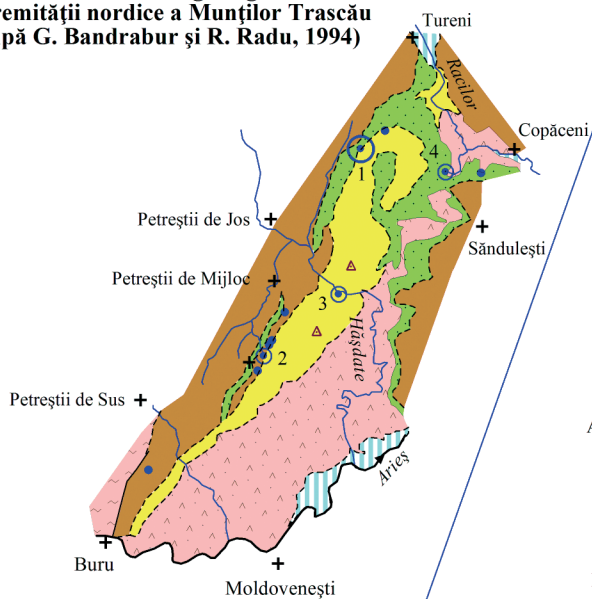
Iancu Orășeanu Fig. 6.1 HARTA HIDROGEOLOGICĂ A MUNTILOR TRASCĂU (Legenda in fig. 1. 6)
