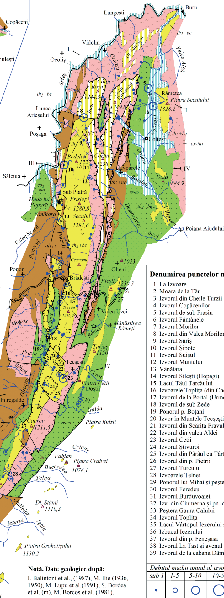
Iancu Orășeanu Fig. 6.1 HARTA HIDROGEOLOGICĂ A MUNTILOR TRASCĂU (Legenda in fig. 1. 6)
