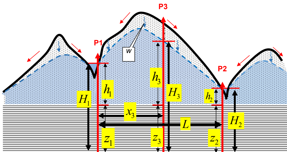
Fig.2. Secțiune pentru calculul modulului de infiltrare ( w )
